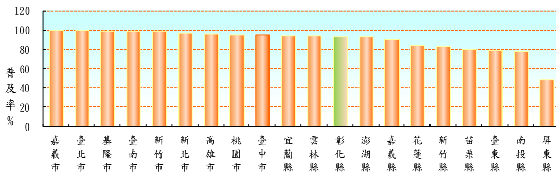
圖三 104年底臺灣地區各縣市自來水供水普及率
