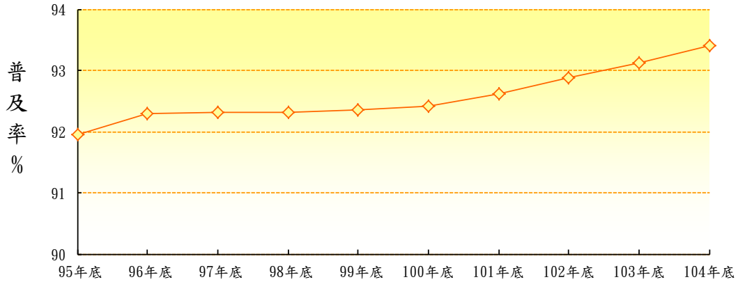
圖一 彰化縣歷年自來水供水普及率
